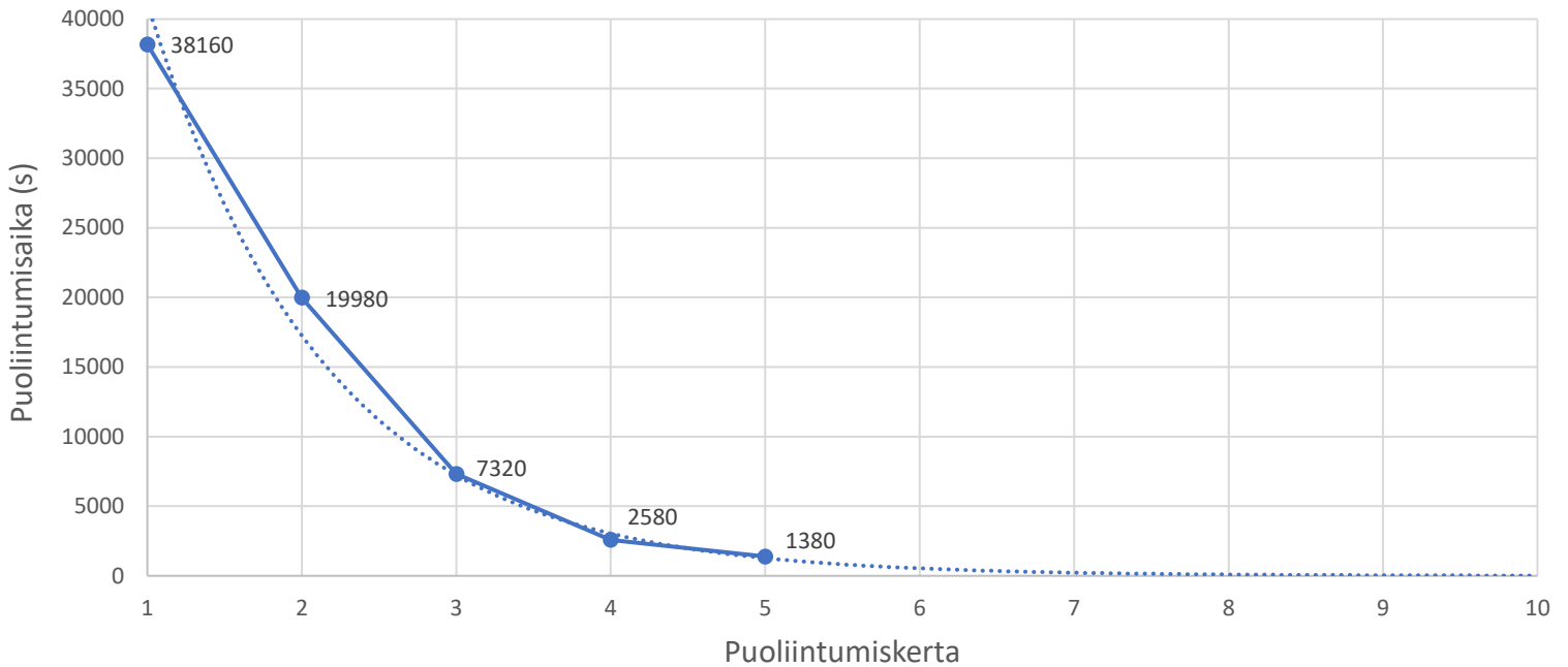
Kuvaaja 1. Kuparin puoliintumisaika havainnollistettuna
